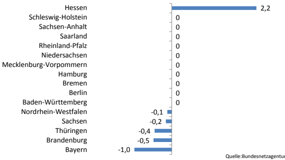
Deponie-, Klär- & Grubengas: Zubau 2014 in MW
